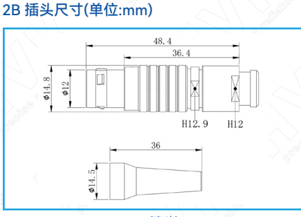
FGG(直头)
