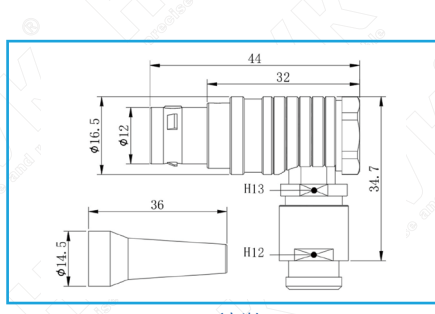
FHG(弯头)
